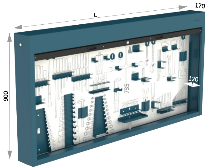
SERIE 110 1 L=1000-1300-1500-1800-2000
