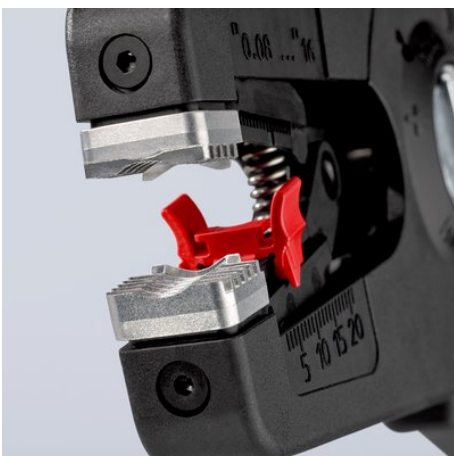
Abrazadera de sujeción acanalada semicircular para un mejor agarre que sujeta prácticamente cualquier material de aislamiento en su lugar
